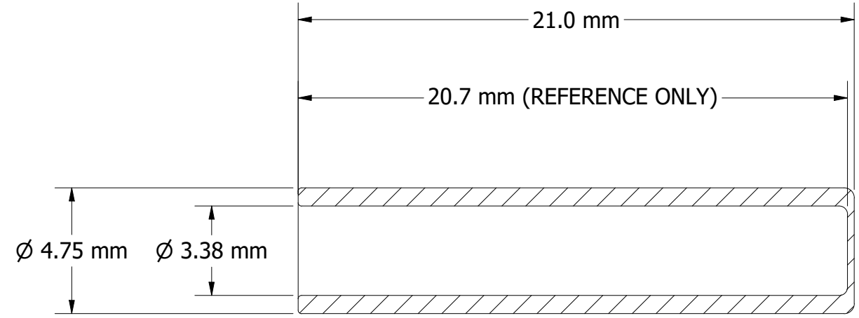
SECTION A-A SCALE 5 : 1
