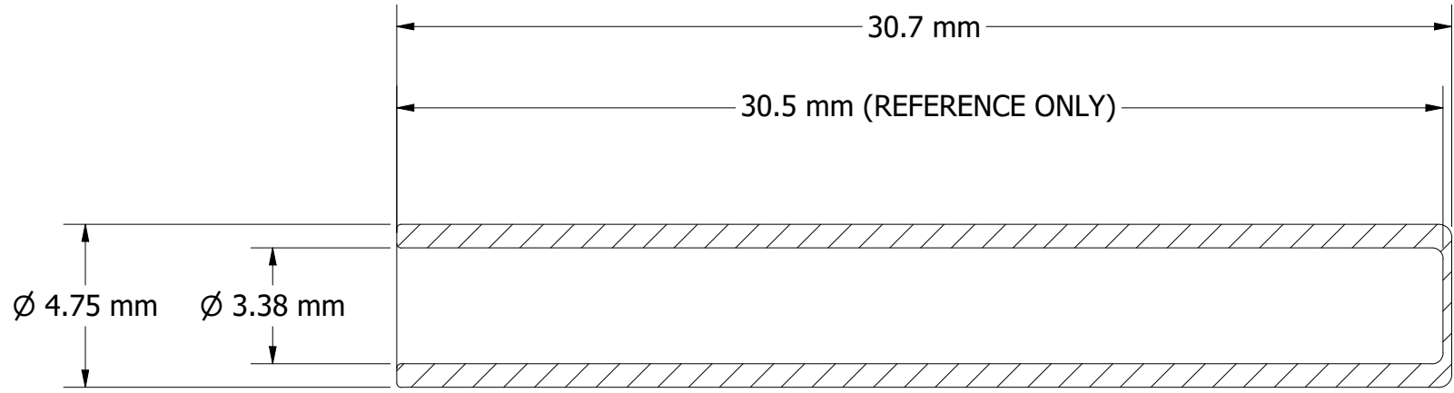
SECTION A-A SCALE 5 : 1
